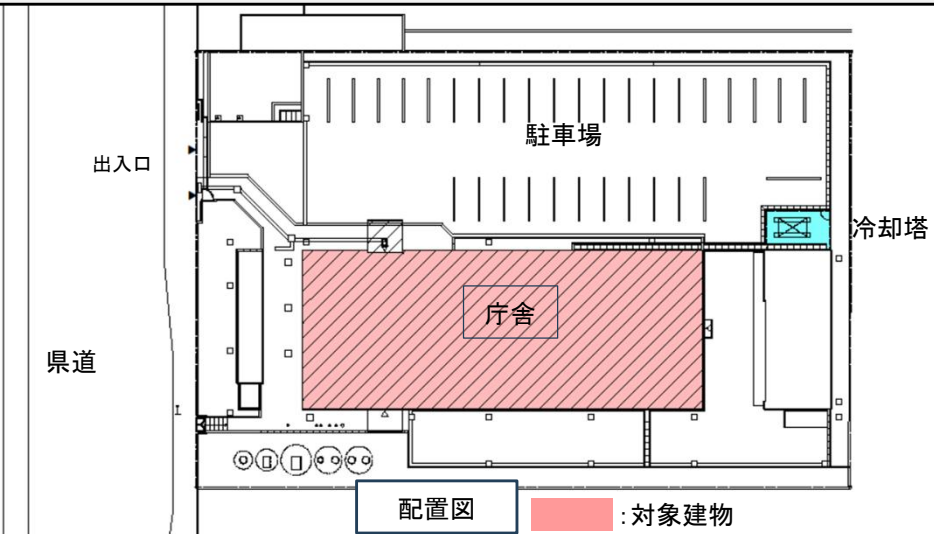
(工事概要図)
