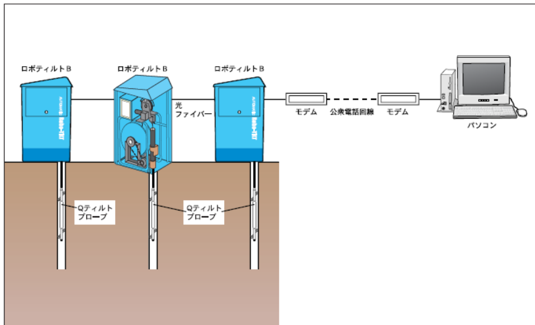
自動観測機器（ロボティルト）及び孔内傾斜計プローブ設置の概念図
