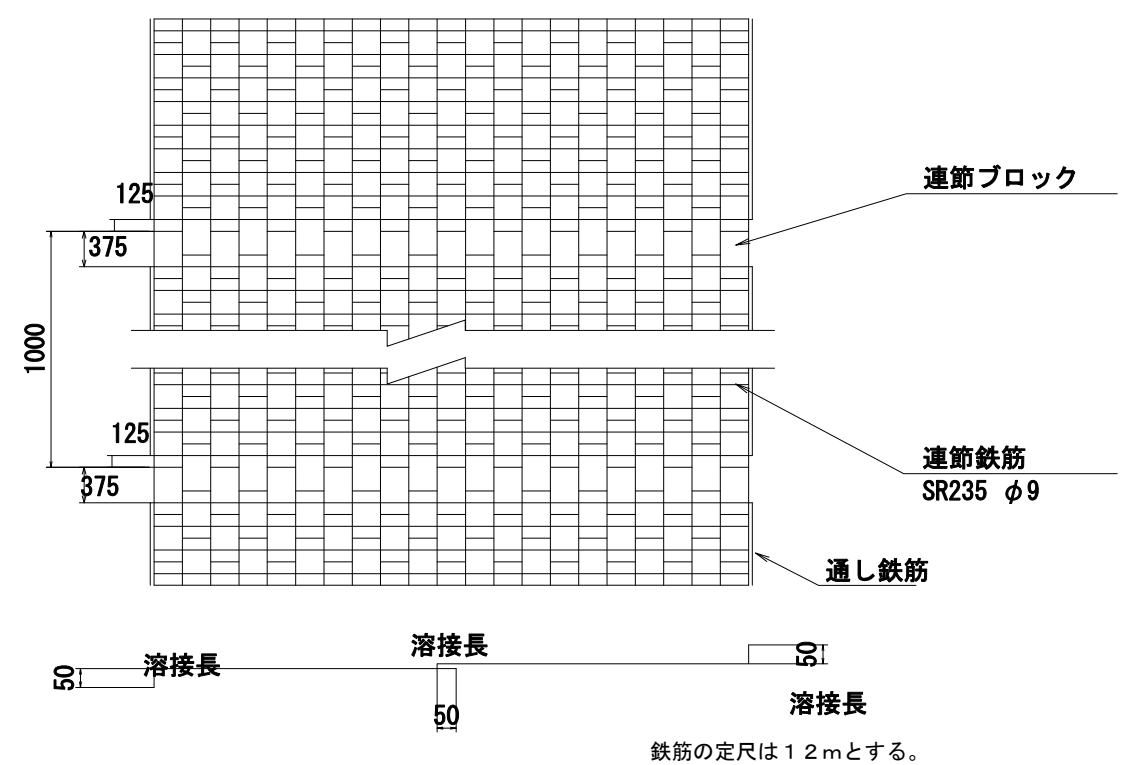
連節ブロック張 S=1:20
