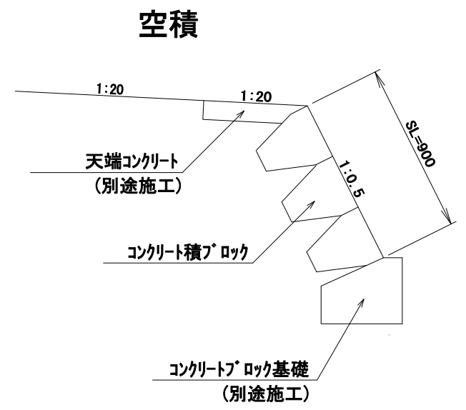
コンクリートブロック積 S=1:20
