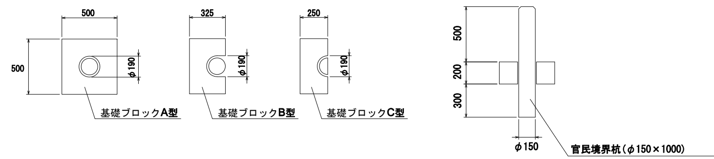
境界杭 S=1:20
