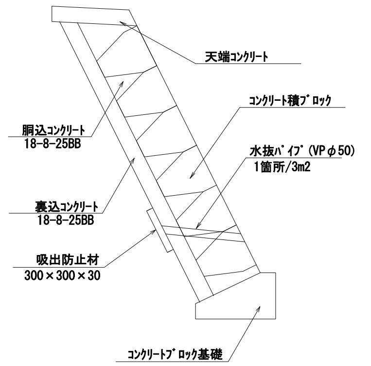
練積(参考図)
