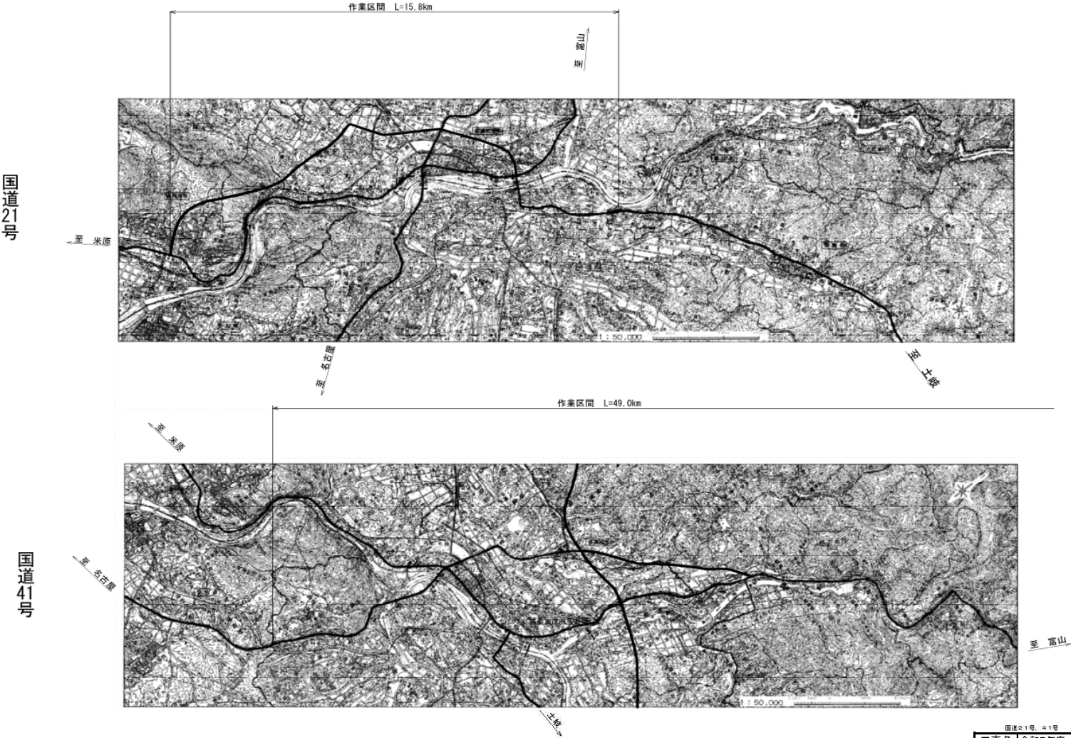
位置図 1
