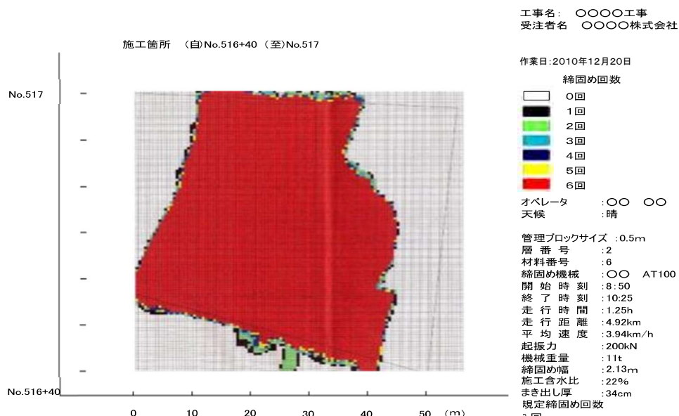
締固め回数分布図例（管理ブロックサイズ 0.50m）
