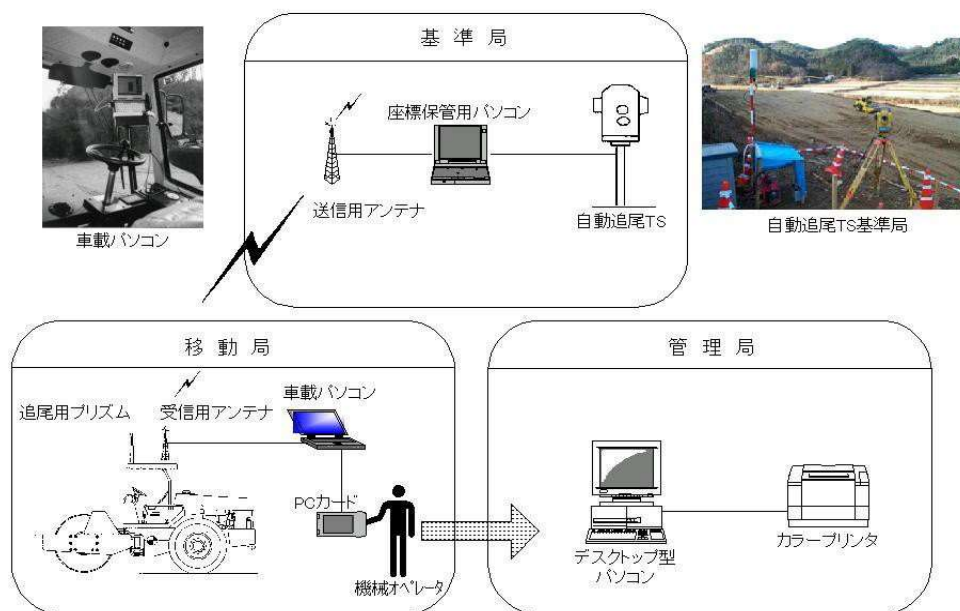
TSを用いた締固め回数管理システム（例）
