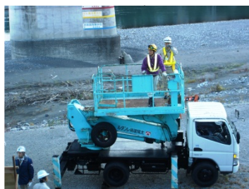
珍しいロッカー支承
