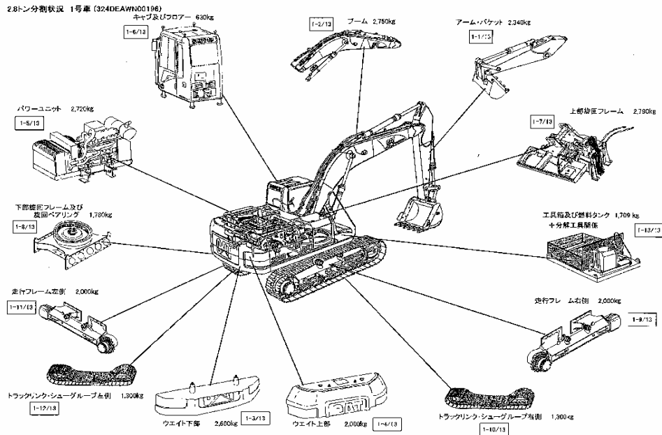
無人化施工バックホウ分解パーツ
