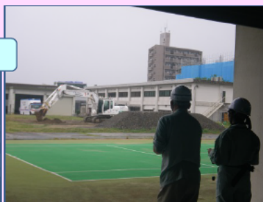
無人化施工バックホウ操作体験
