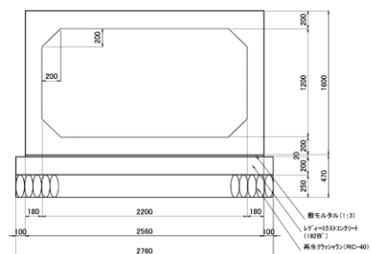
標準断面図
