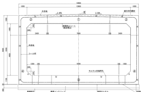
標準断面図
