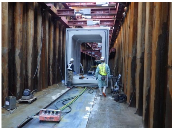
写真①横引き状況
