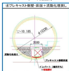
トンネル断面図
