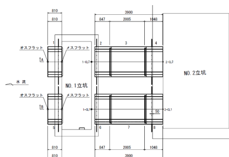
平面配列図
