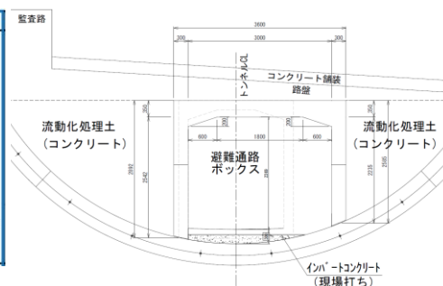
プレキャスト断面図
