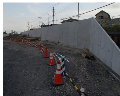
プレキャスト部材設置完了
