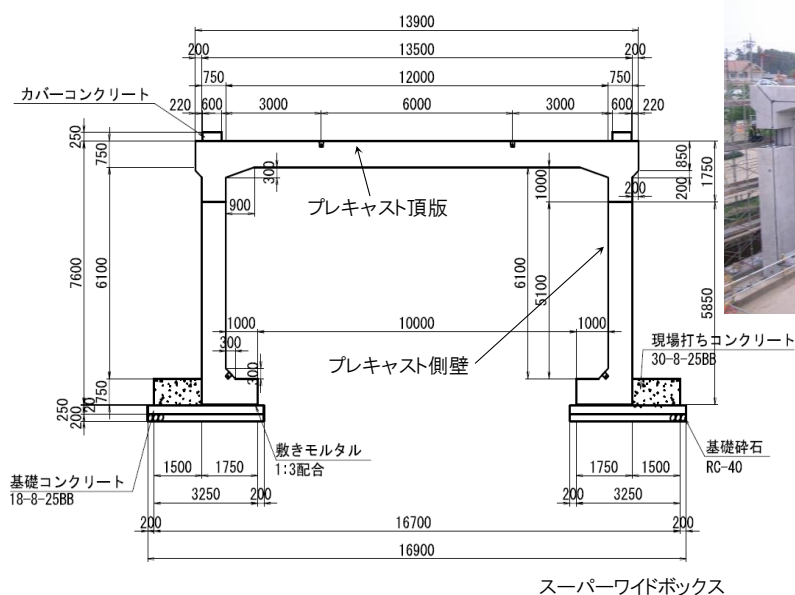
断面図
