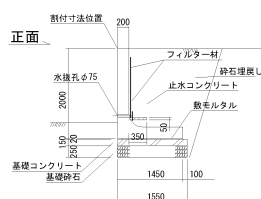
プレキャストL型擁壁コーナー部
