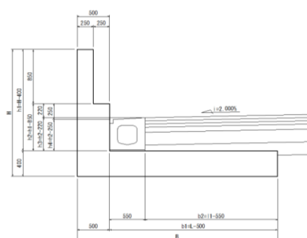
外回り剛性防護柵
