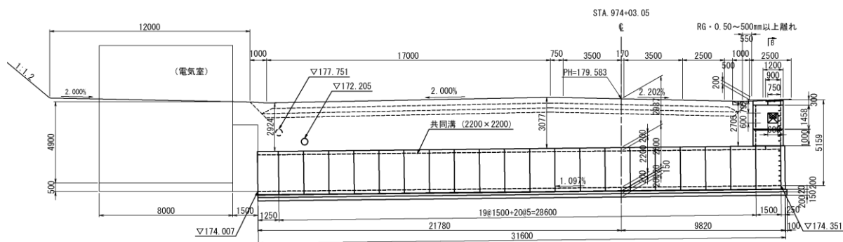
縦 断 図 S=1:250
