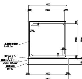
断面図 S=1:40
