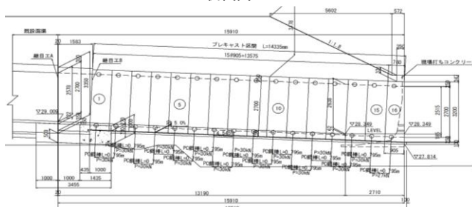
側面図
