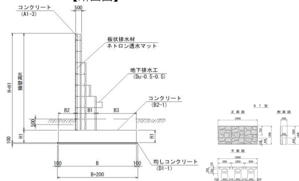
【断面図】
