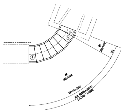
平面図 S=1:100
