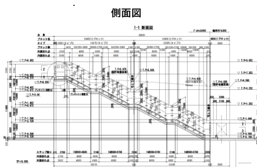
プレキャスト部材搬入
