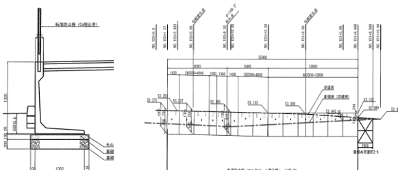
断面図 S=1.40 (S=1:200) L=25m 展開図 S=1:100 (L: 50) S=1:200 (L: 100)
