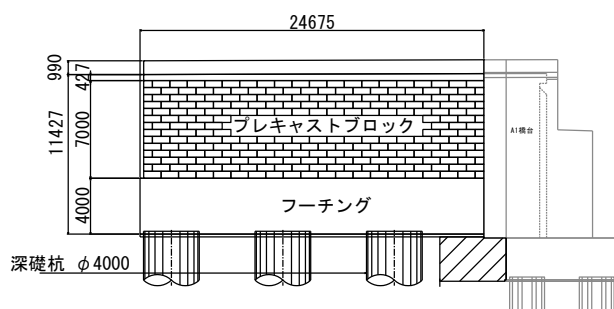
図-1 正面図
