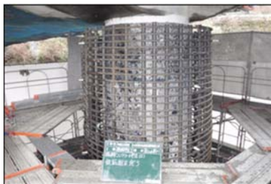
耐震工事例
