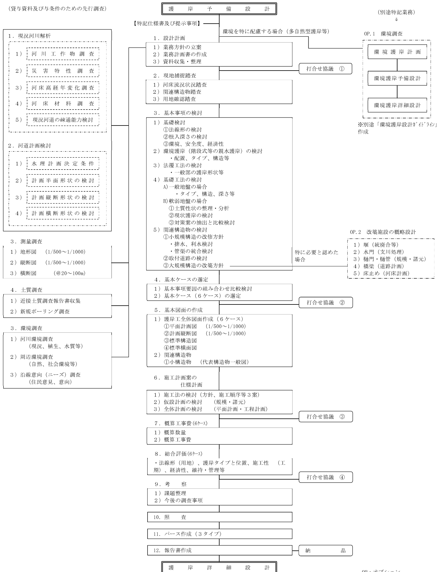
護岸設計フローチャート（1）
