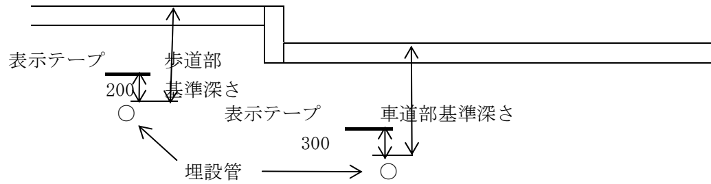
図2-5 埋設深
