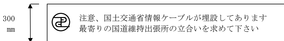
図 2-4 埋設テープ
