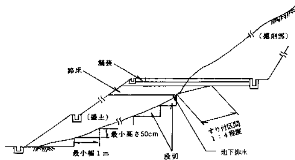
図 2-2 盛土基礎地盤の段切
