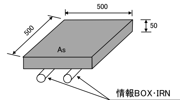
図 1-1 試掘標準図
