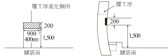
図 10-6-1 覆工厚変化箇所の刻示標準図
