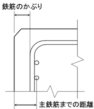
図 1-3-1 鉄筋のかぶり
