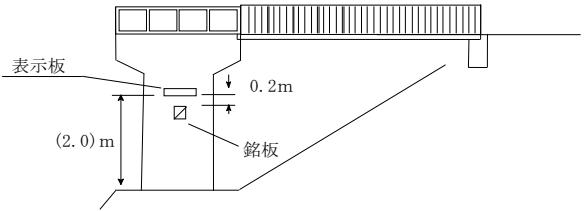
図3－1 樋門の銘板及び表示板の取付け場所
