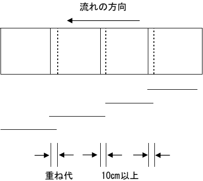
図 1－1 吸出し防止シートの重ね代
