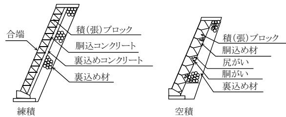
図2-5 コンクリートブロック工
