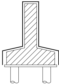
図－３ 橋梁下部
