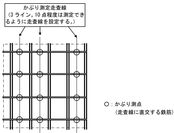
図 5 かぶりの測定
