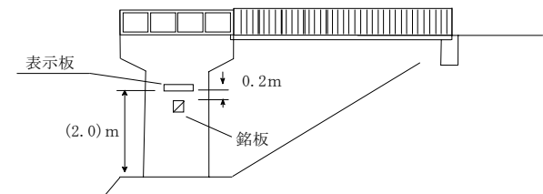
図 3-1 樋門の銘板及び表示板の取付け場
