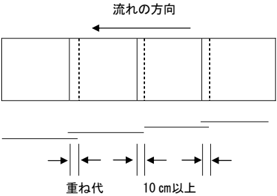
図 1-1 吸出し防止シートの重ね代
