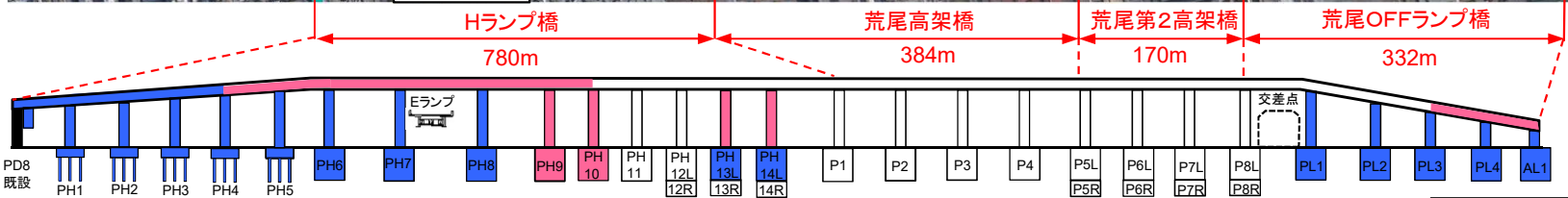
⑤Hランプ橋(PH14→PH8方向)
