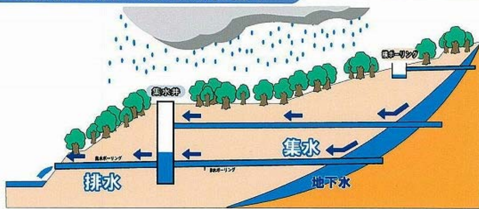
集水井・横ボーリングの仕組み
