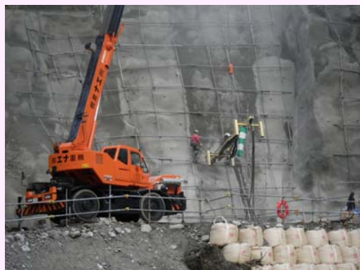
鉄筋挿入工 (スカイドリル工法) 岩盤へ鉄筋を串刺しにして 補強しました。
