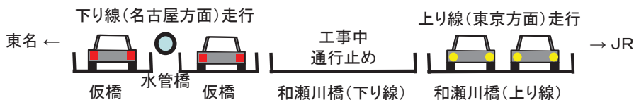
国道1号 和瀬川渡河箇所 断面イメージ(東京側から名古屋側を見る)
