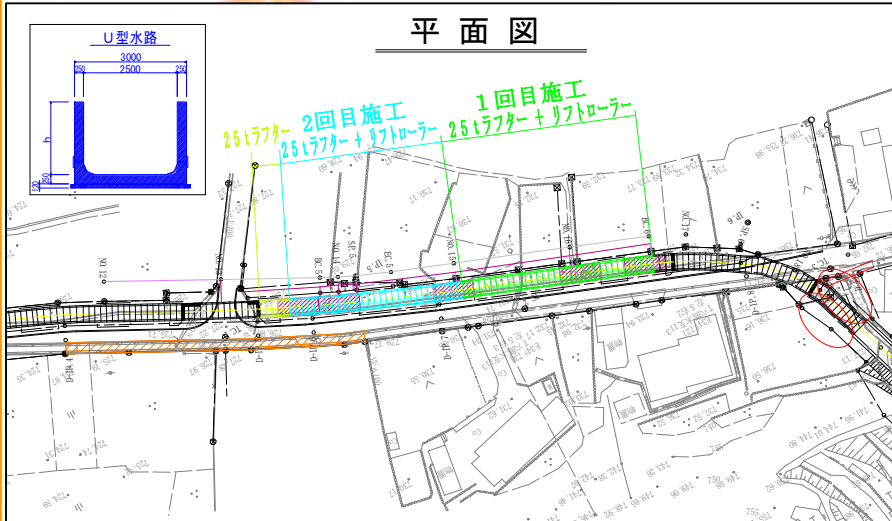
リフトローラーでの水路運搬設置状況事例
