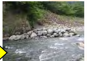
(写真2)袋詰玉石を空洞部に (写真3)重機にて巨石を並べる (写真4)完成状況(全景)
