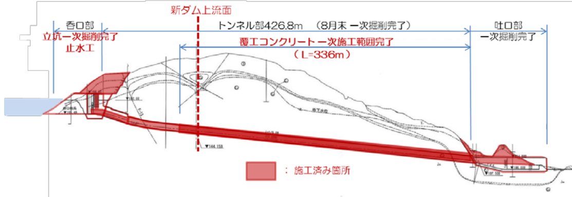
転流工事進捗状況 (令和元年8月末時点)
