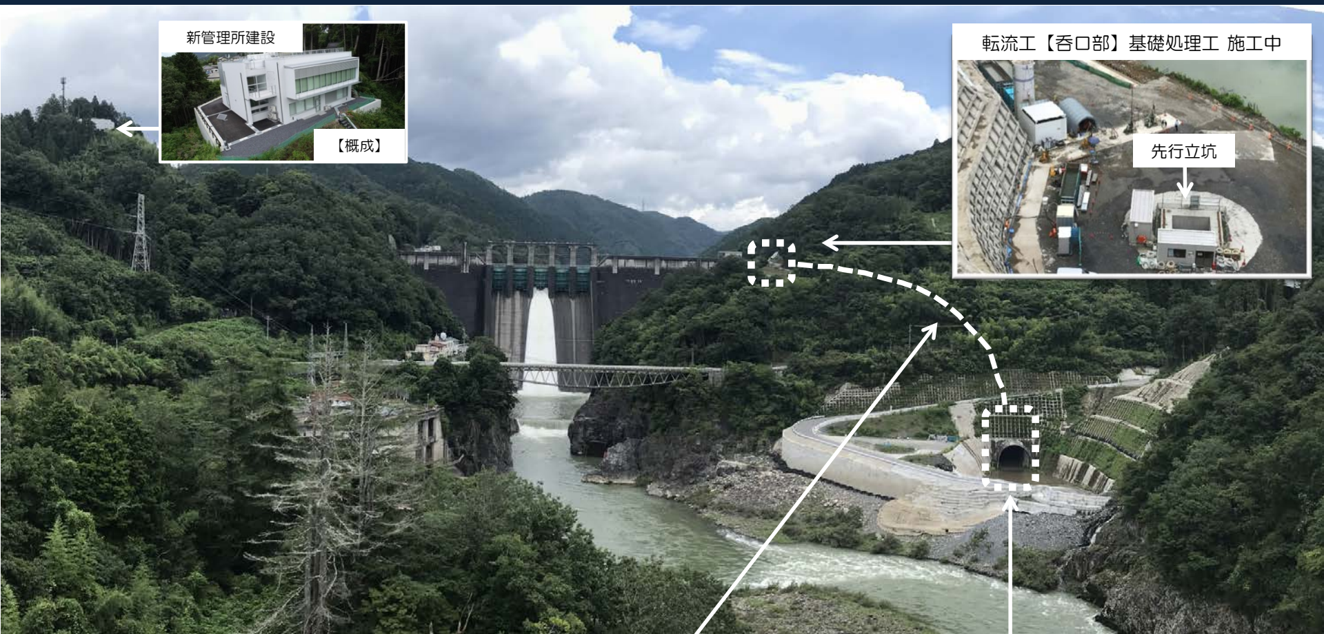
転流工事進捗状況 (令和元年8月末時点)
