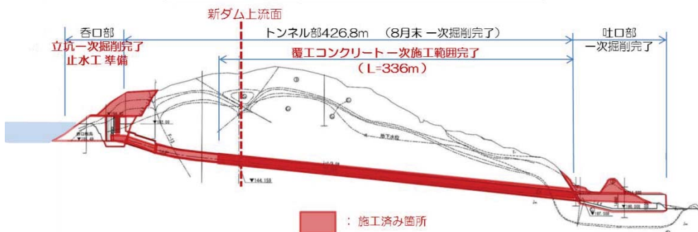
転流工事進捗状況 (平成31年3月末時点)
