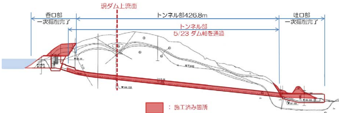
転流工事進捗状況 (平成30年6月末)
