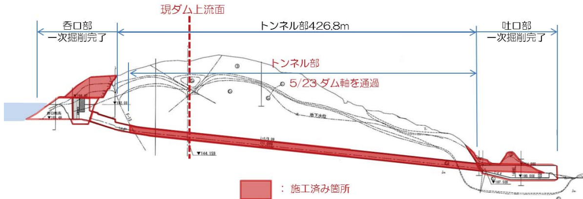
転流工事進捗状況 (平成30年5月末)
