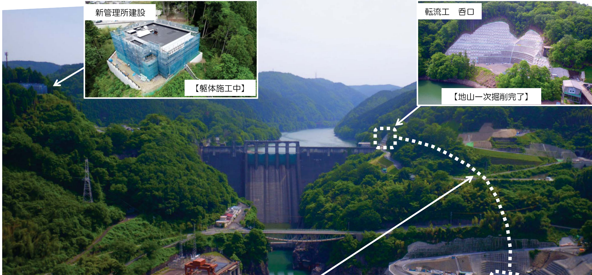
転流工事進捗状況 (平成30年5月末)
