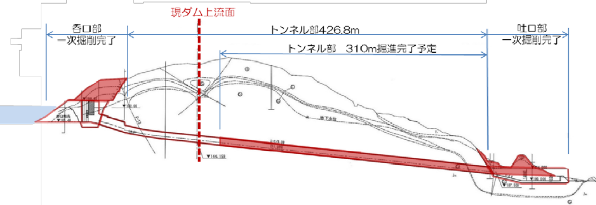
転流工事進捗状況 (平成30年4月末)
