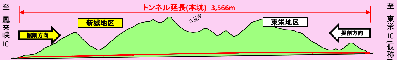
トンネル縦断面図
