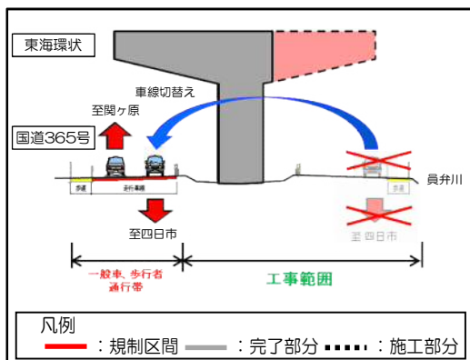
車線切替えイメージ
