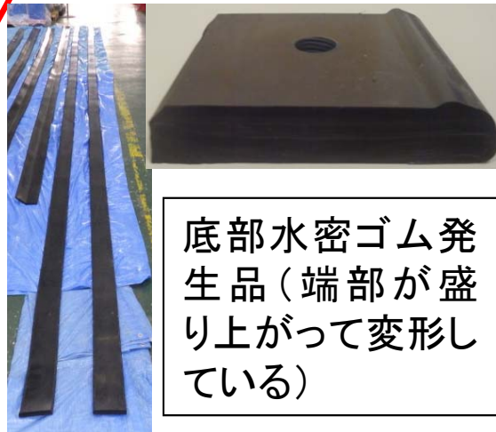
底部水密ゴム
