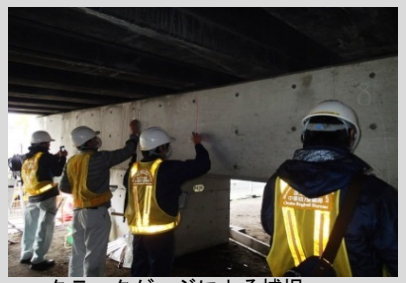
クラックゲージによる捕捉
