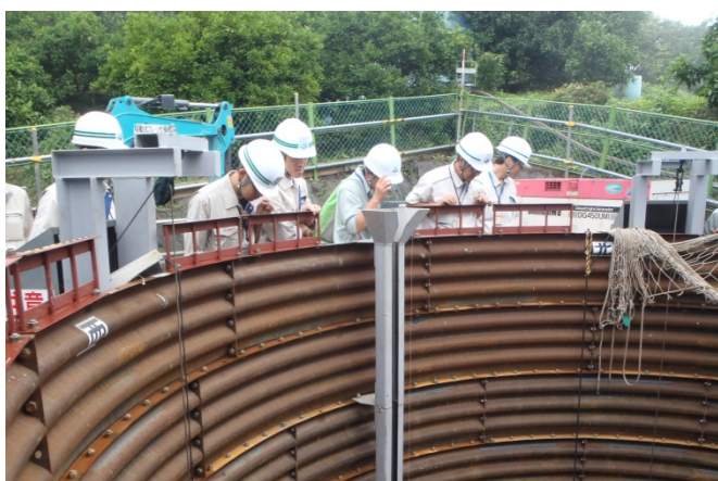
深礎杭工施工現場の説明
