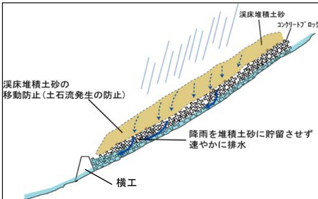
▲ブロックスクリーン工の構造
